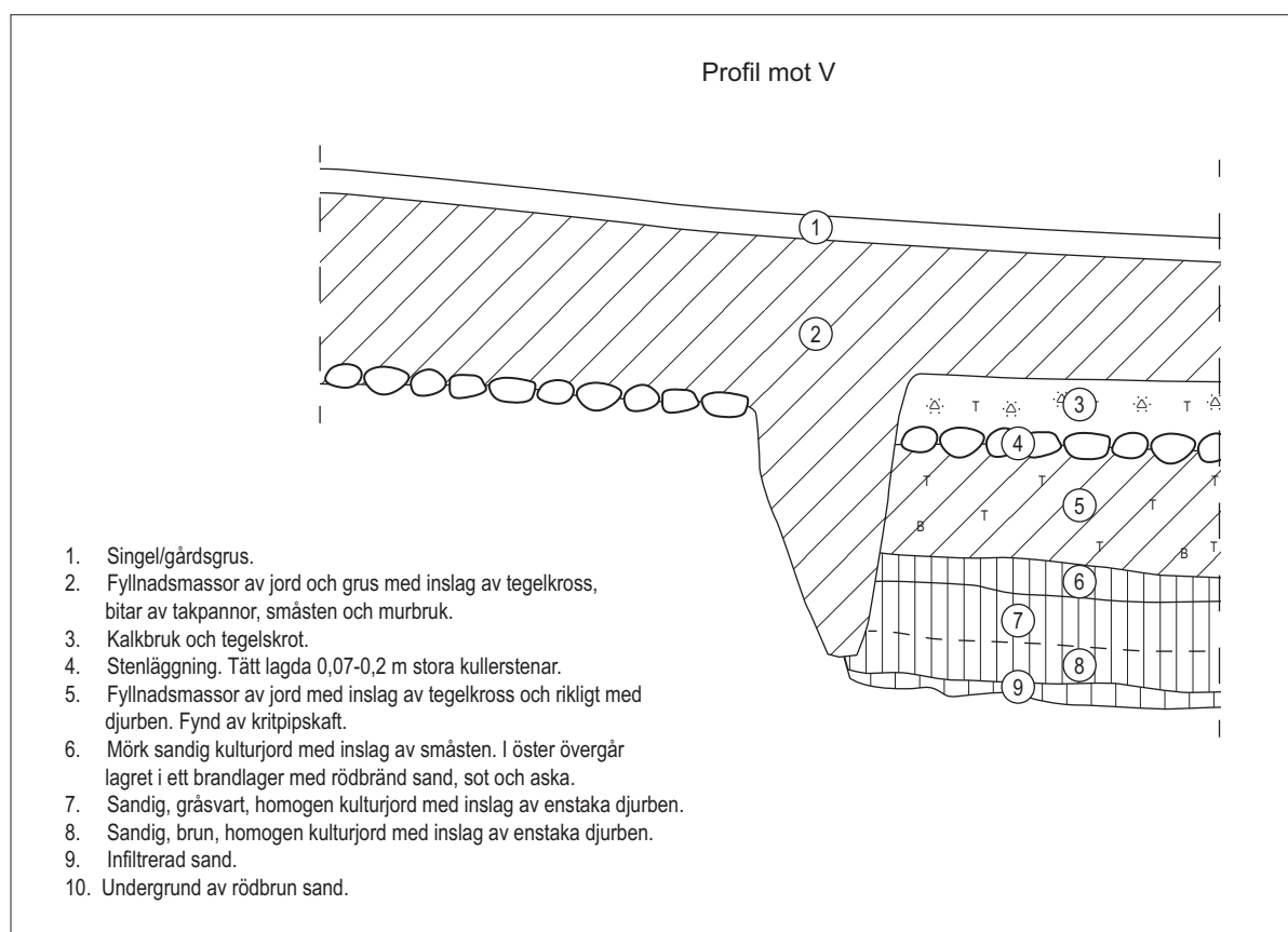
Figur 7. Schaktprofil mot väster. Skala 1:20.
