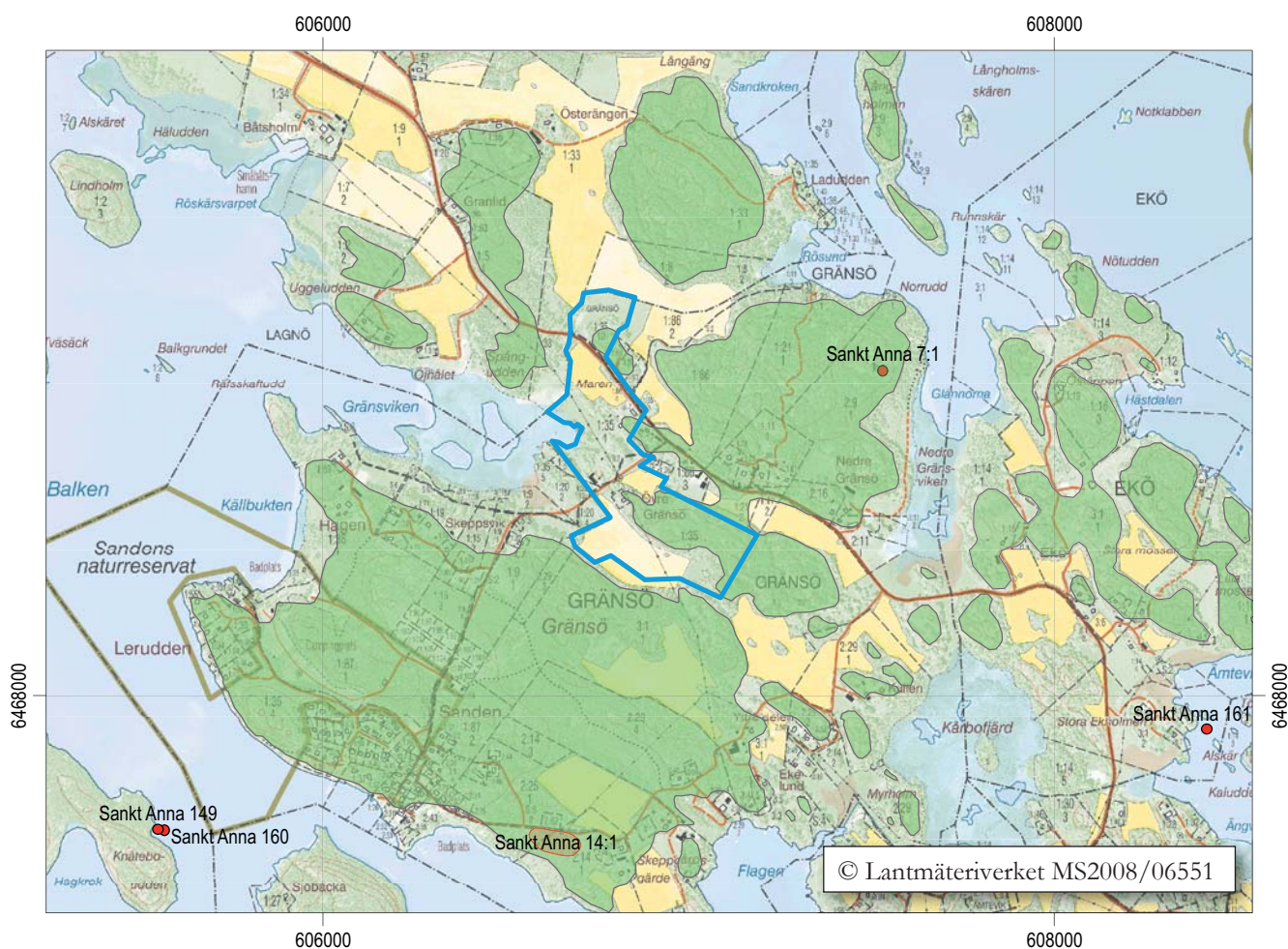
Figur 3. Utredningsområdet som det ter sig med en 5 m högre havsnivå, då endast de gröntonade områdena låg över havsytan. Skala 1:20 000.
