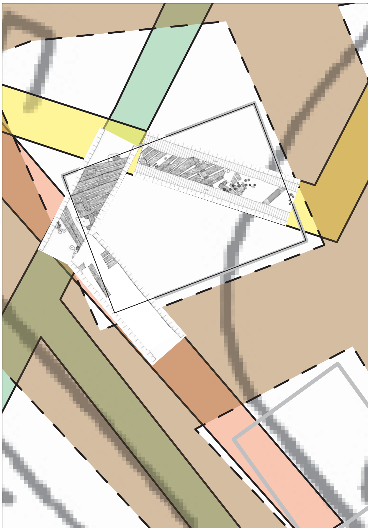
Figur 11. Rekonstruktion av byggnad (A4) utifrån tre arkeologiska undersökningar vid Vintervadsplan. Teckenförklaring se fig 10. Skala 1:100.
