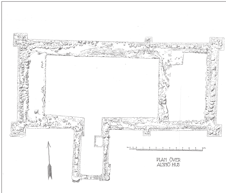
Figur 10. Planritning över Alsnö hus (Thordeman 1920).
