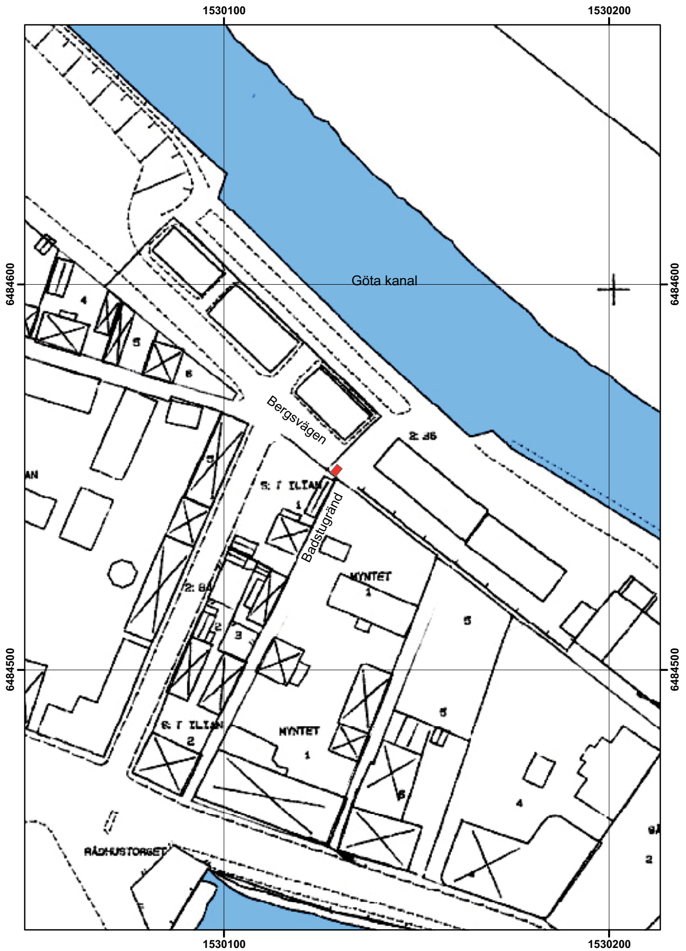
Figur 4. Utdrag ur Adresskartan över Söderköping, med schaktet i Bergsvägen markerat.
