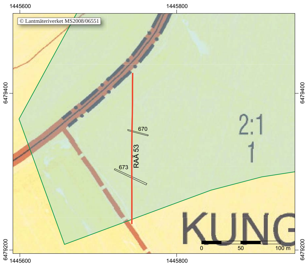
Schaktplan. Skala 1:2 500.
