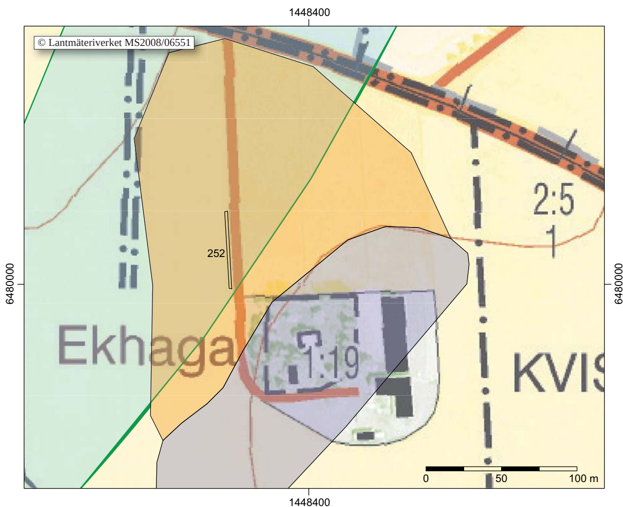
Schaktplan. Skala 1:2 500.
