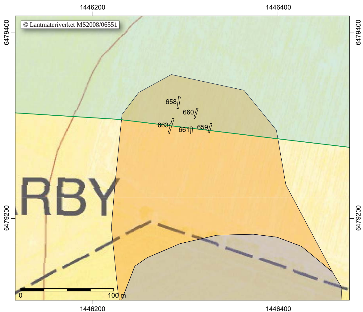
Schaktplan. Skala 1:2 500.
