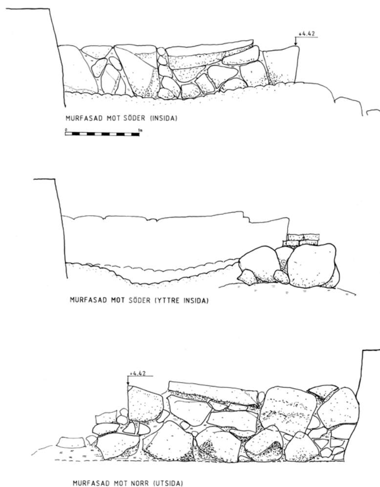
Figur 18. Muren i profil. Skala 1:50.
