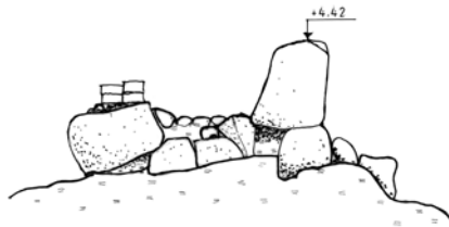
Figur 15. Muren i profil. Profilen är ritad där muren brutits av vid tidigare grävning. Den inre muren har varit påbyggd med tegel av vilket rester fanns kvar. Skala 1:50.
