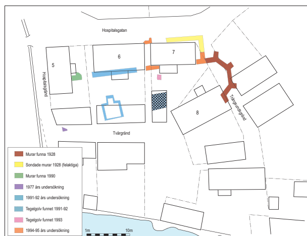
Figur 6. De hittills påträffade murarna i Hospitalsstugekvarteren. Svart = murar påträffade 1991-95, grått = tidigare kända murar, vitt = antagna mursträckningar.
